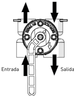
Funcionamiento normal Sistema de descalcificación
